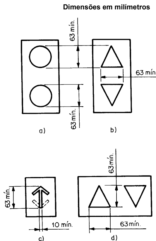
Figura 10 - Setas indicadoras de sentido nos pavimentos
