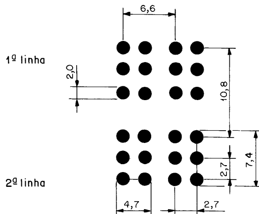
Figura 2 - Arranjo de quatro células braille, distribuídas duas em cada linha
