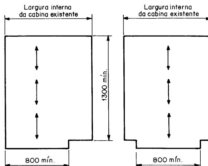
Figura 13 - Arranjo para acomodar uma cadeira de rodas
