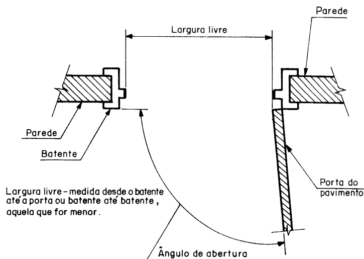
Figura 12 - Largura livre da porta de eixo vertical (porta batente)
